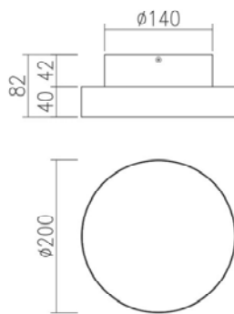
Technische Zeichnung
